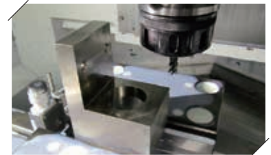
部品加工
