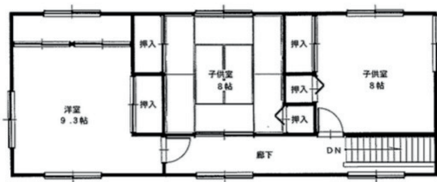
平面詳細図 2階
