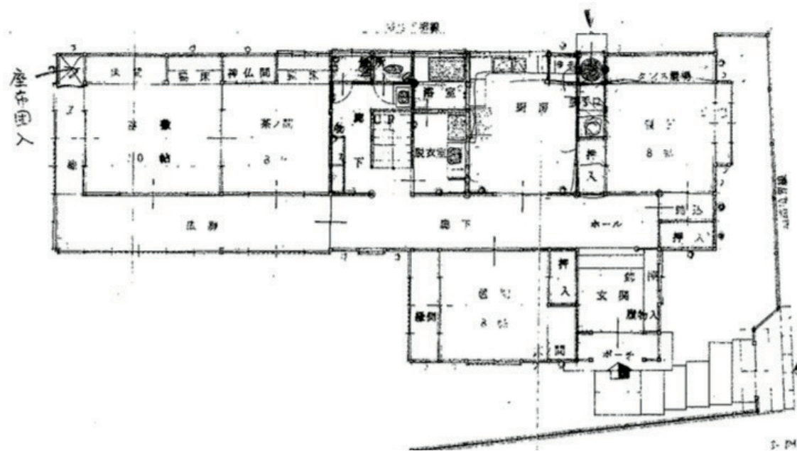
《間取り図 1 階》
