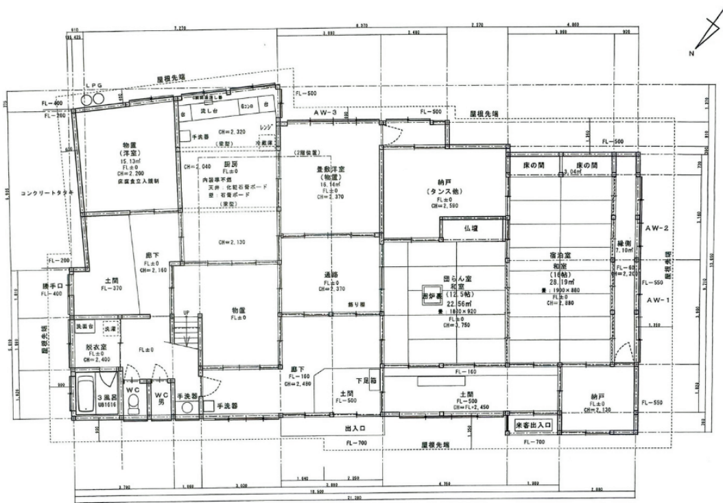
1階平面図
