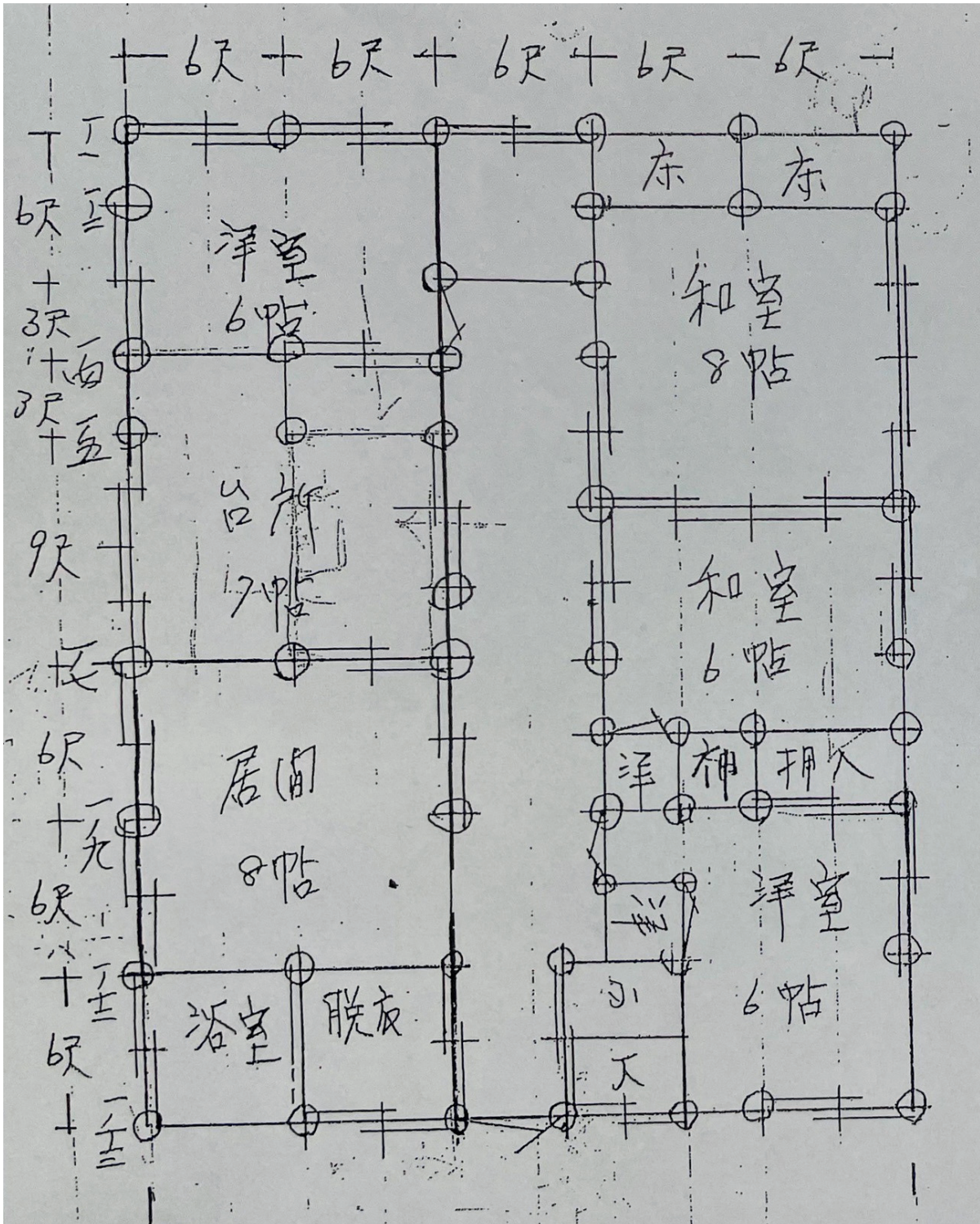
<間取り図>
