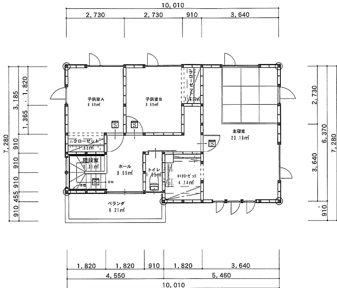
平面詳細図 2階
