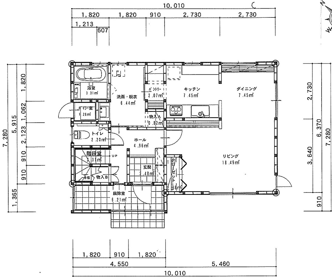
平面詳細図 1階
