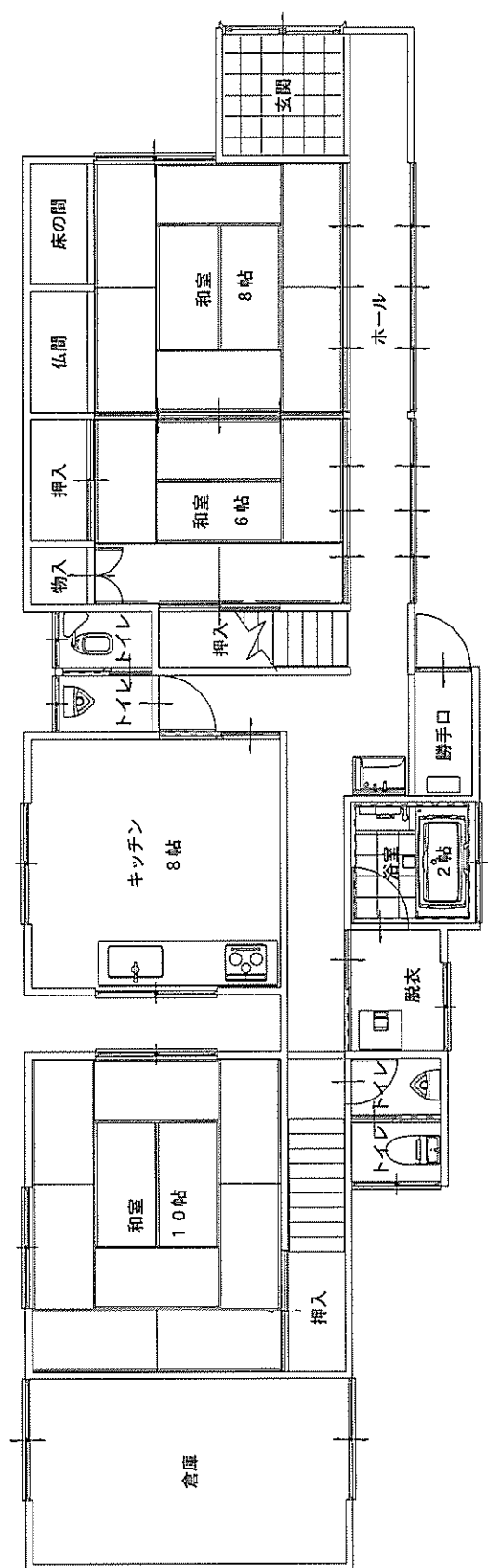
平面図 1 階
